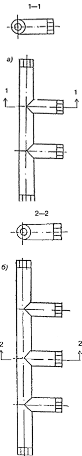
Рисунок 1 - Стальной распределительный коллектор
